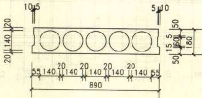
YKBXX9X (YKBaXX9X)
