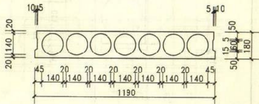
YKBXX12X (YKBaXX12X)
