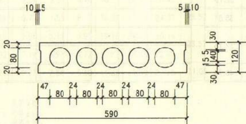
YKBXX6X (YKBaXX6X)
