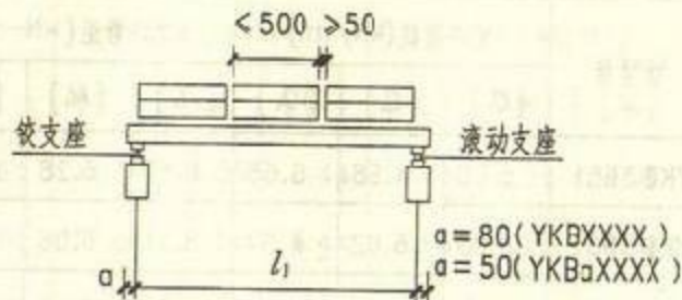
图 1 加荷简图
