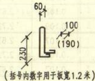
吊钩简图
