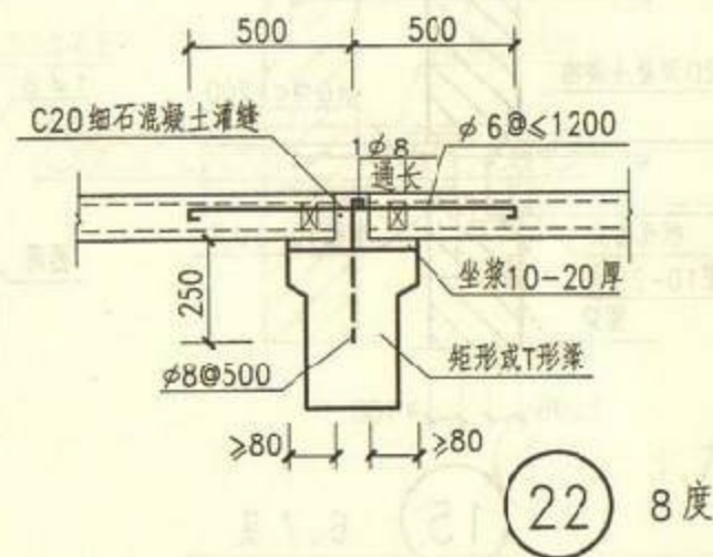
板端连接构造详图(五)
