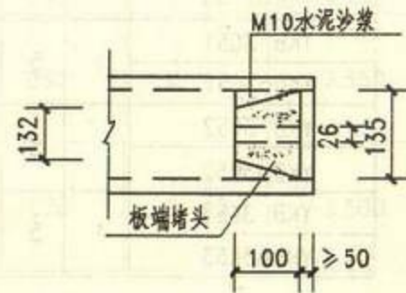
板端堵头 (二)
