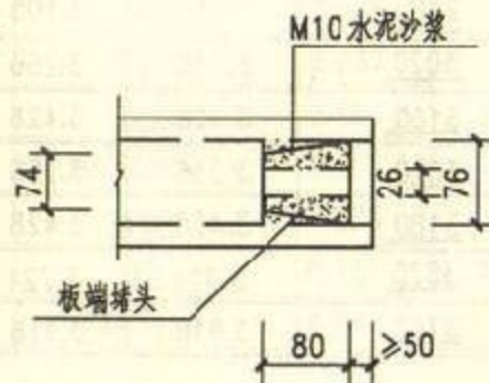
板端堵头 (一)
